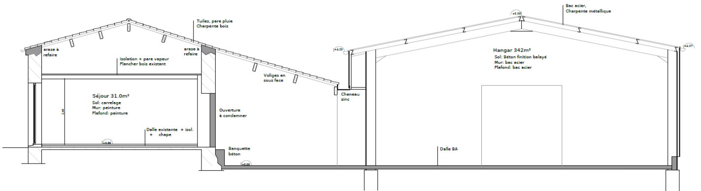
Figure 4 - Coupe bâti habitation et agricole - ferme du Pointeau. Echelle 1/50
