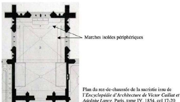
Emmarchement au droit des vitrines d'exposition de la salle du « Trésor »
