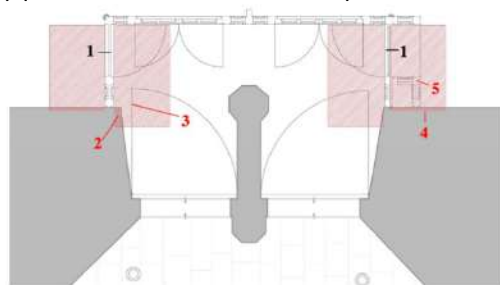
Plan du tambour au droit du portail de la Vierge (en rouge les aires de manœuvre réglementaires de part et d'autre des portes)
